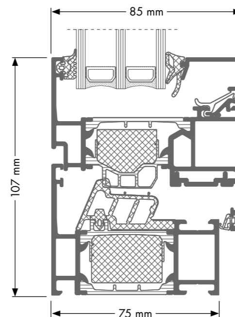
SL 75, Blendrahmen, Flügelprofil
